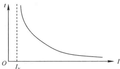
图 1-7 熔断器的反时限保护特性
