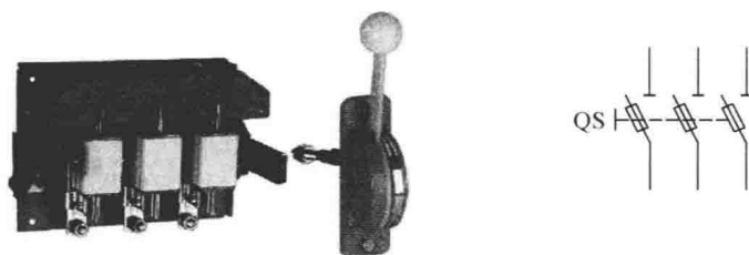
图 1-5 HR 型熔断器式刀开关实物图及图形符号
