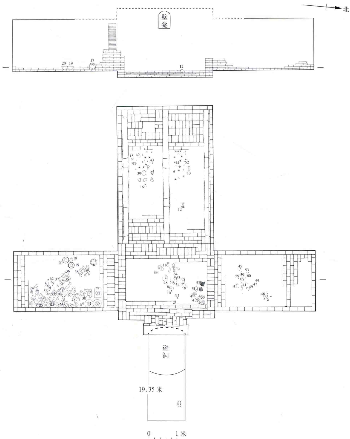
图二 M1 平、剖面图
