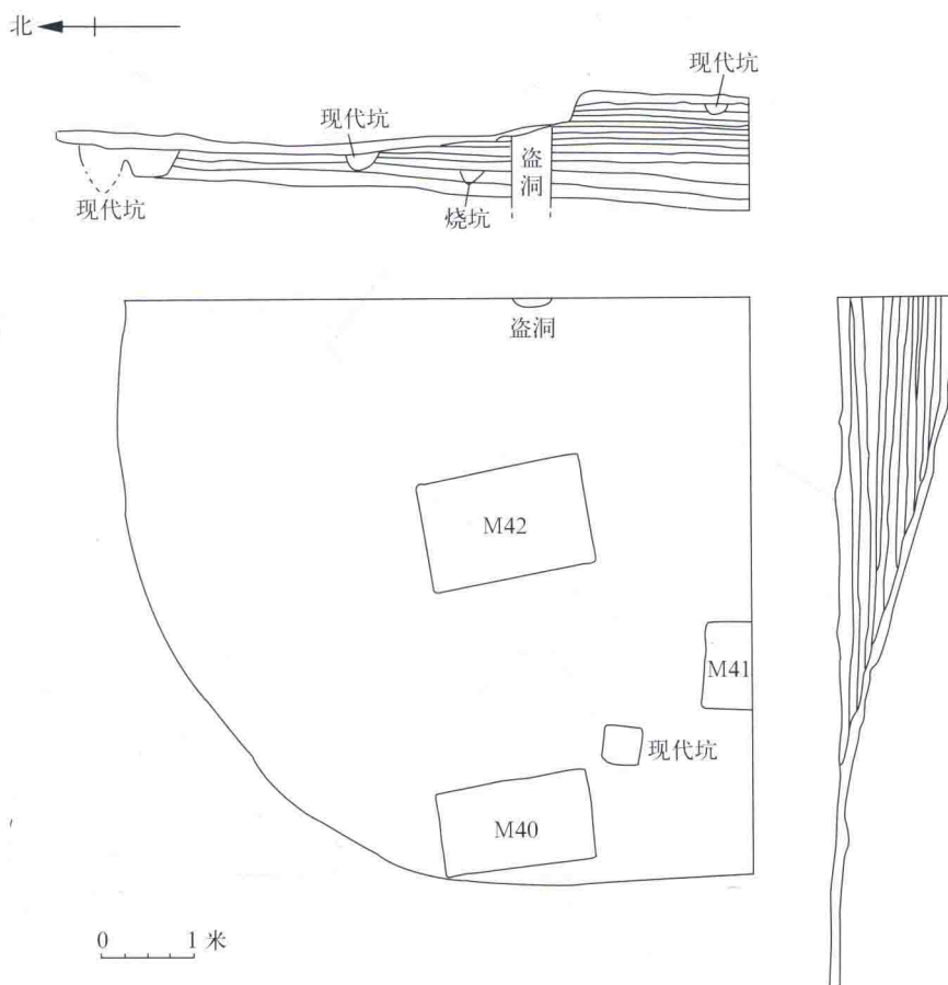
图四 M1 封土解剖图
