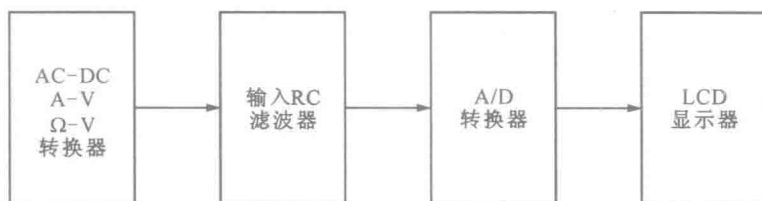
图 1.4 数字万用表原理框图
