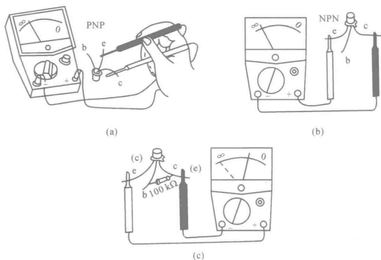
图 1.2 三极管电极判别方法
