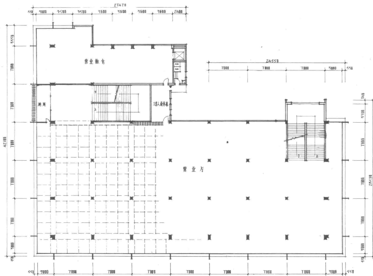
二层平面图
