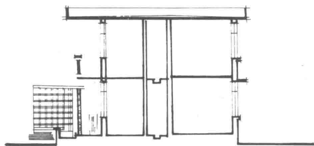
I—I 剖面图
