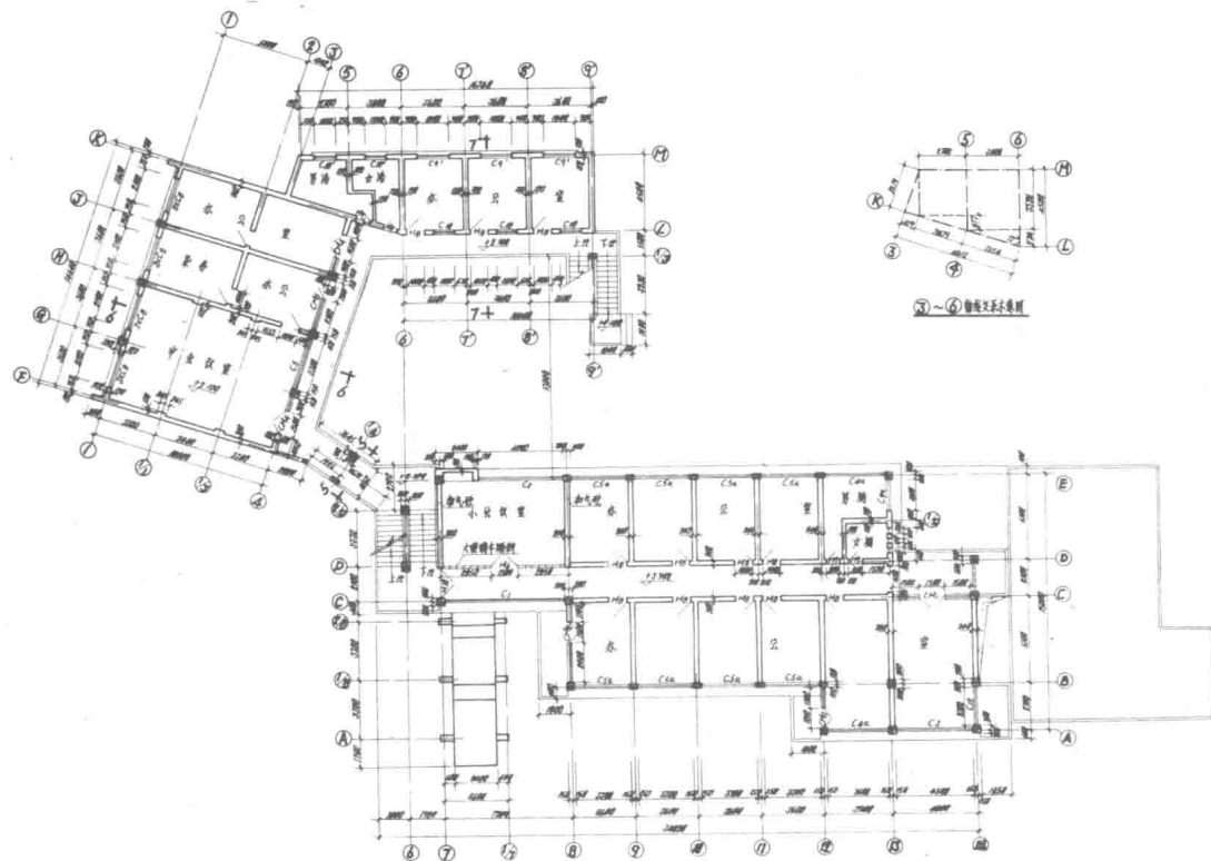
二层平面图
