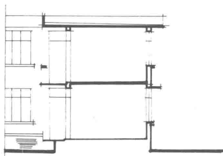
I—I 剖面图
