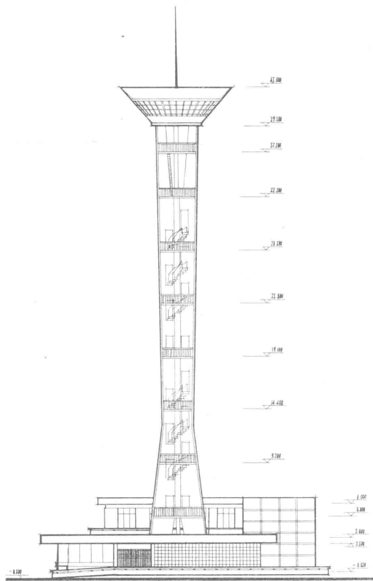
立 面 图
