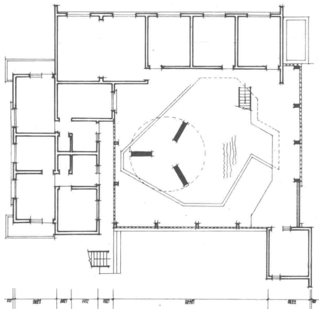
底层平面图
