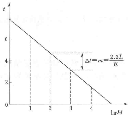
图 1-2 t - \lg H 直线
