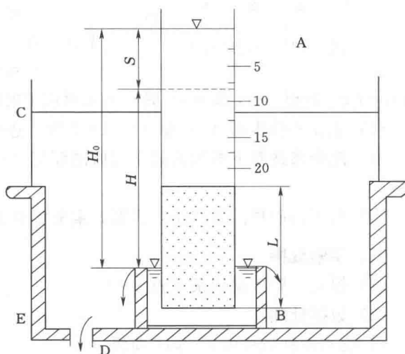
图 1-1 实验装置图
