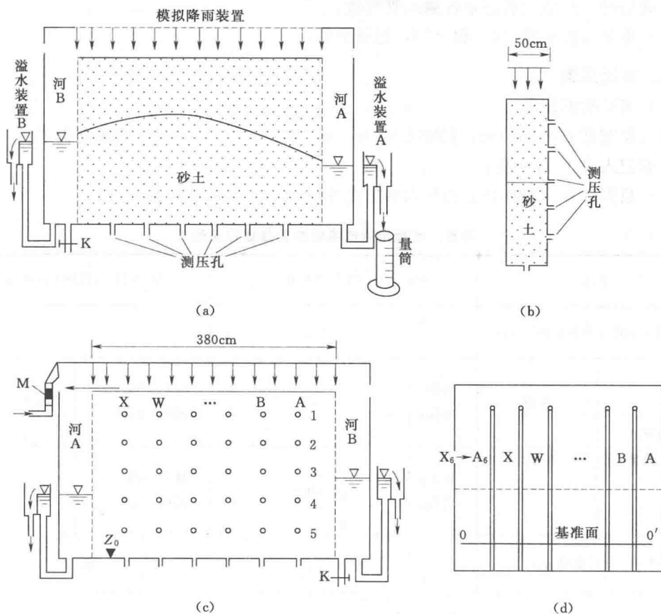
图 1-3 二维渗流实验装置示意图
