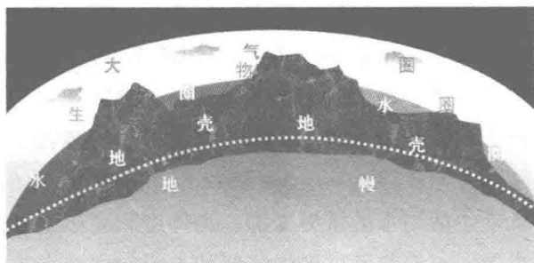
地球圈层
