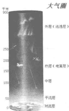
大气圈
