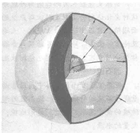
地幔和地核
