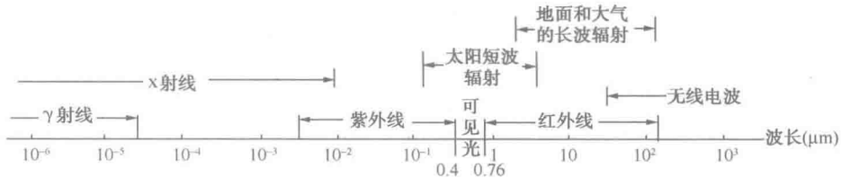
图 1-2 电磁波谱的波长范围
