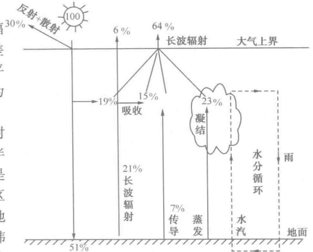
图 1-3 地气系统的热量收支
