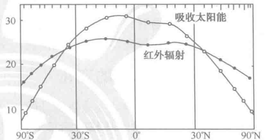
图 1-4 地气系统各纬度辐射收支
