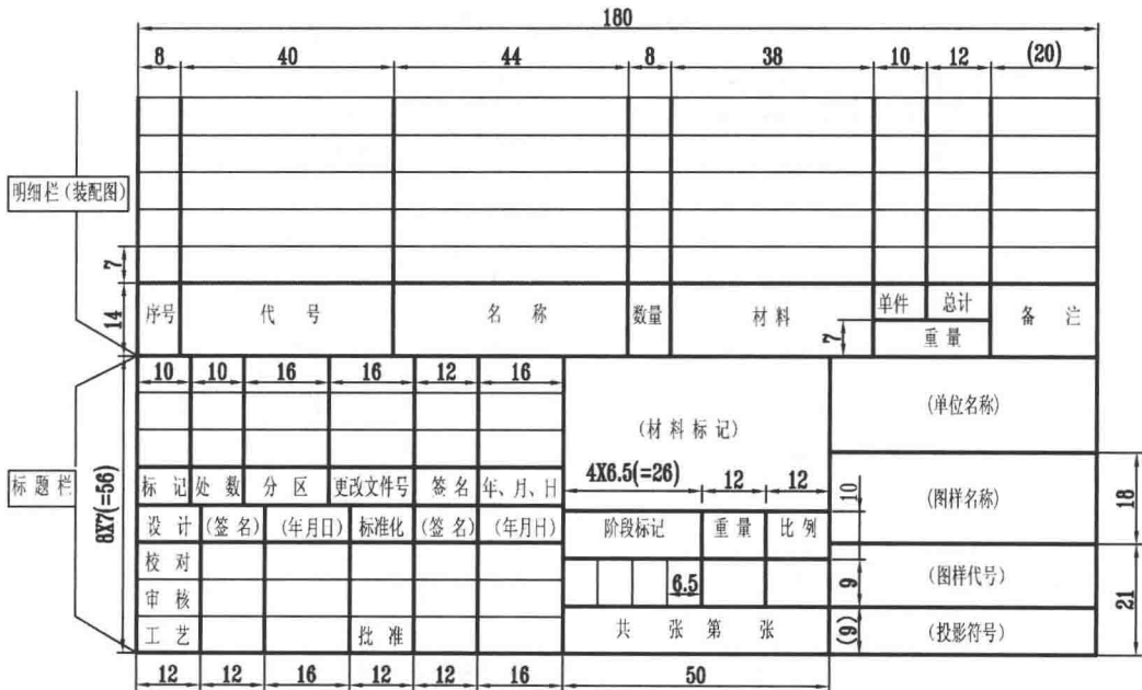
图 1-1 标题栏和装配图中明细表的格式
