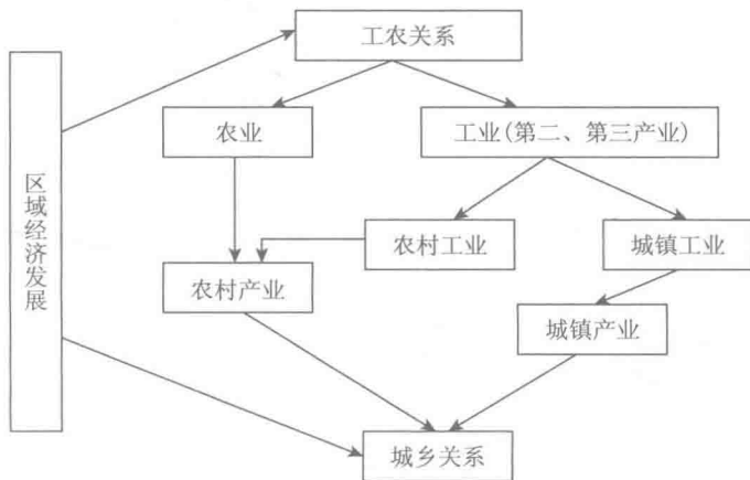
图 1-1 工农、城乡关系发展示意
