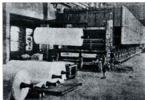
1973年8月，营口造纸厂研制的9号造纸机生产出优质凸版书刊纸。
