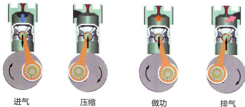
四冲程发动机工作原理图
