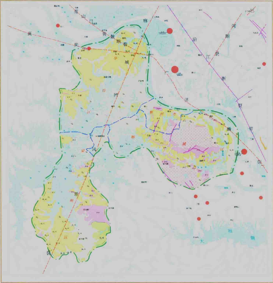
鄂州市地震构造图
