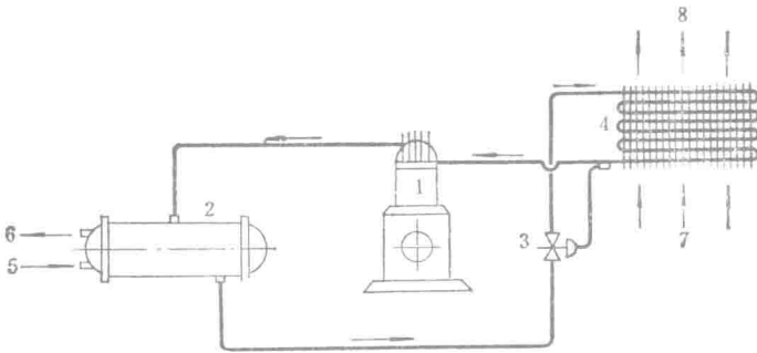
图 0-2 压缩致冷系统
