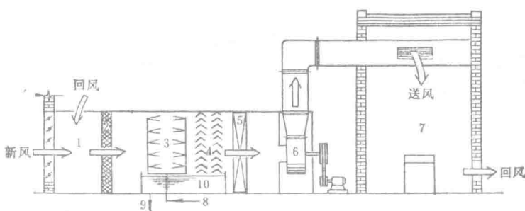
图 0-3 一次回风空调系统
