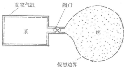
图 1-2 闭口系统
