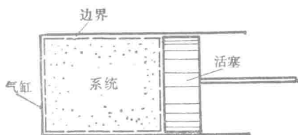
图 1-1 热力系统
