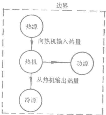
图 1-4 孤立系统
