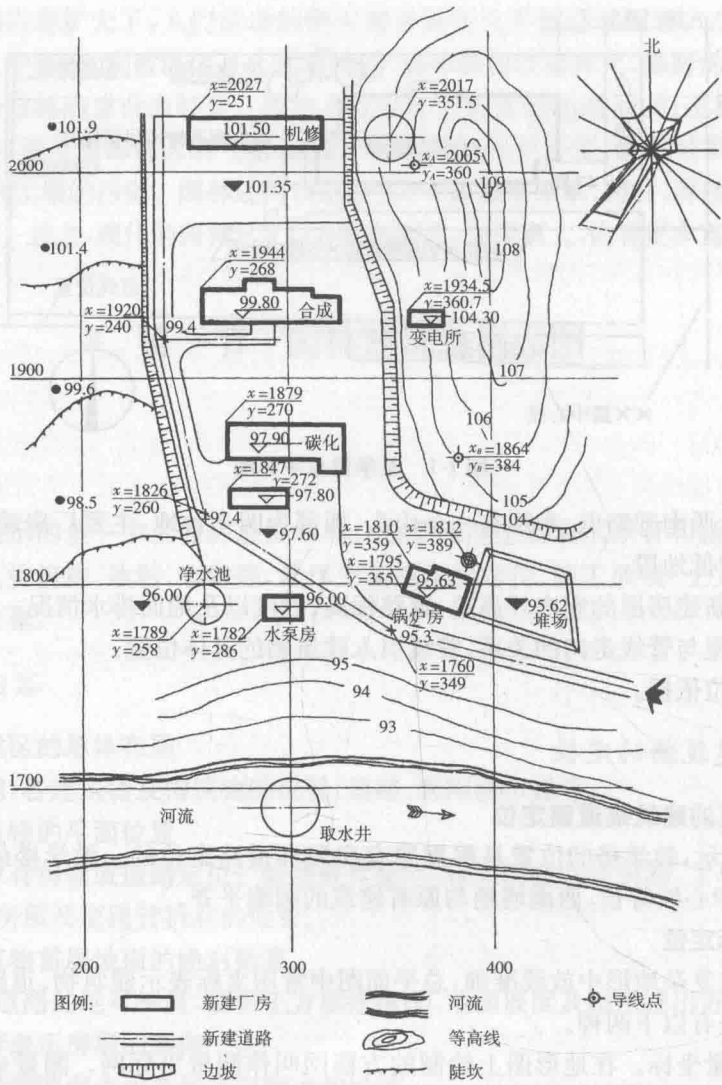
图 1-2 某工厂总平面图
