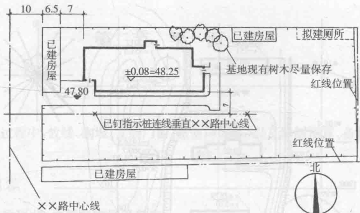
图 1-1 某学校总平面图
