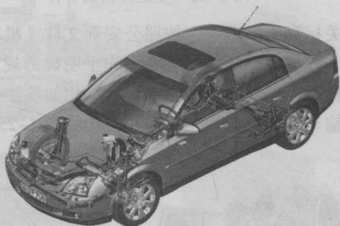
图 1-18 底盘检查
