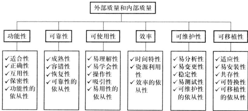
图 1.1 外部质量和内部质量的质量模型
