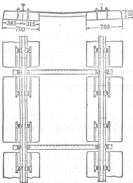
图—5 纵向轨枕轨道
