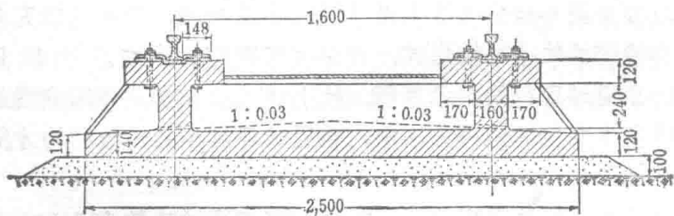
图—3 整体道床轨道
