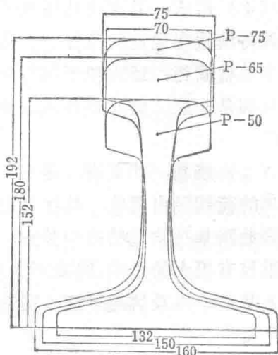
图—2 苏联重型钢轨
