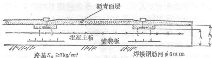
图—4 组合式轨道混凝土整体道床
