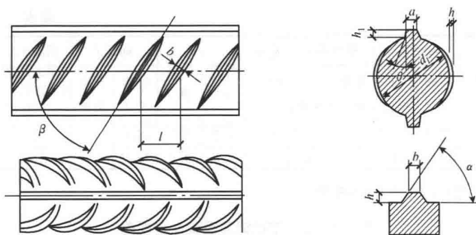
图 1-2 月牙肋钢筋表面及截面形状
