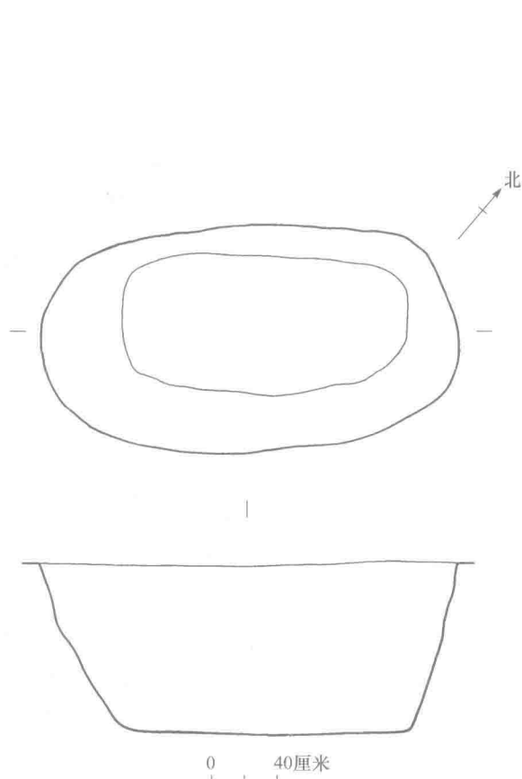
图三九七 IV T1902H419 平、剖面图
