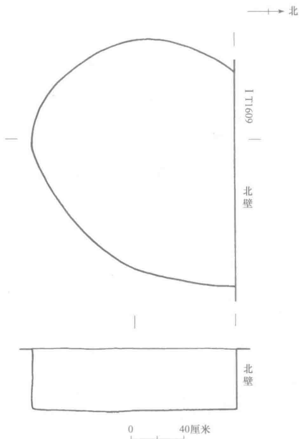
图四〇〇 IV T1609H104 平、剖面图
