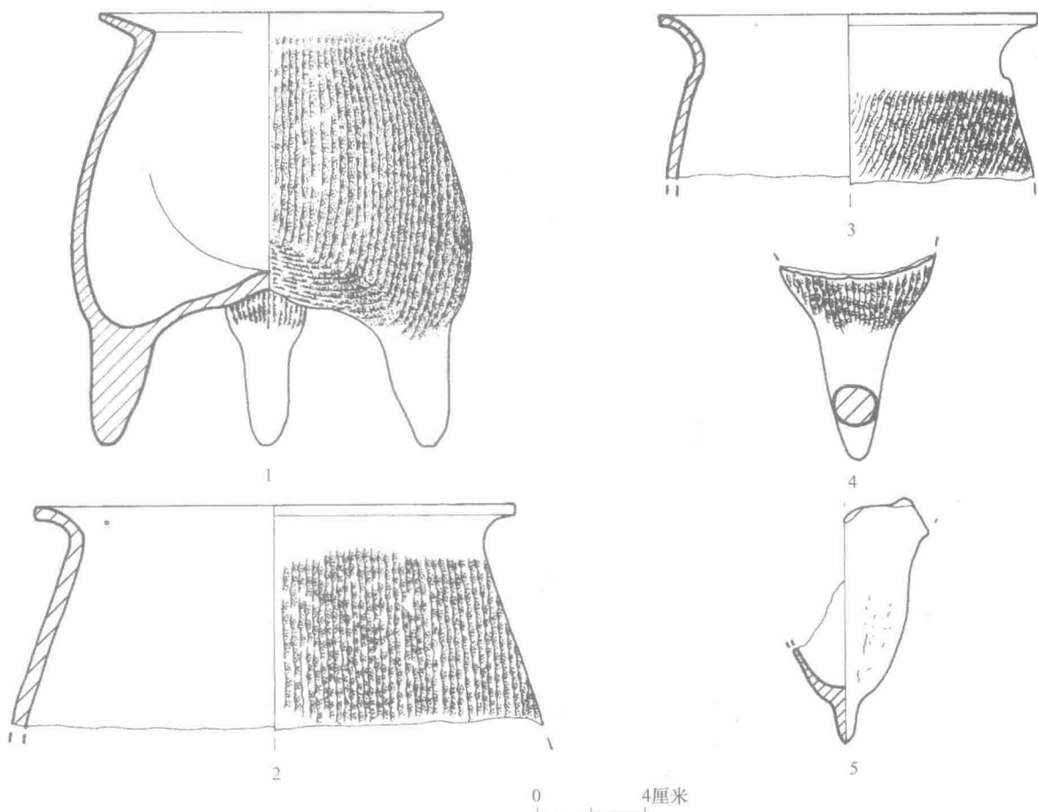
图四〇五 陶鬲、甗足
