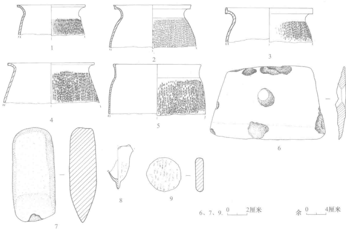
图三九五 IV T0505H658 出土器物
