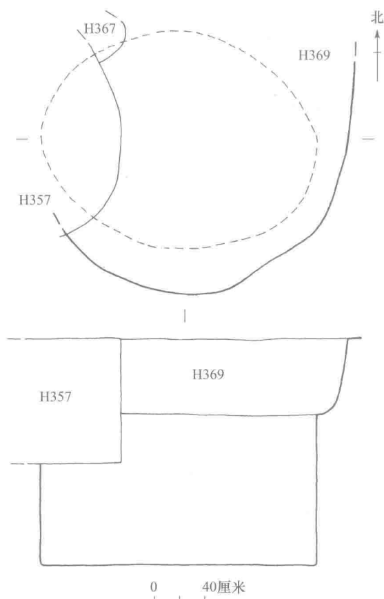
图三九六 I T0707H371 平、剖面图
