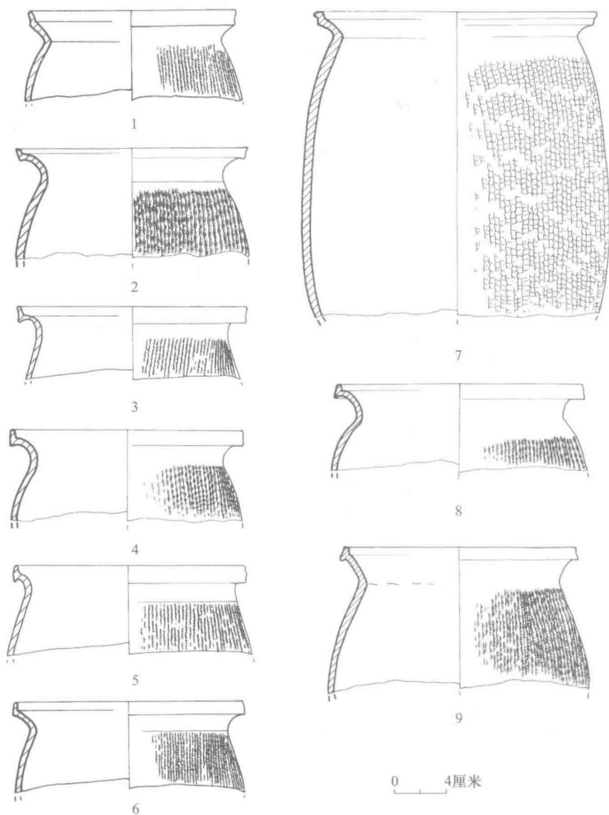
图四〇六 陶深腹罐
