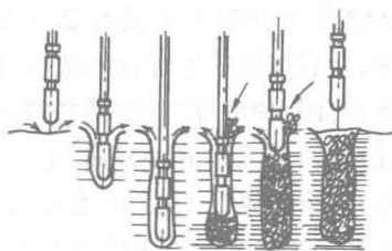
图 1-2 振冲法施工顺序稳固
