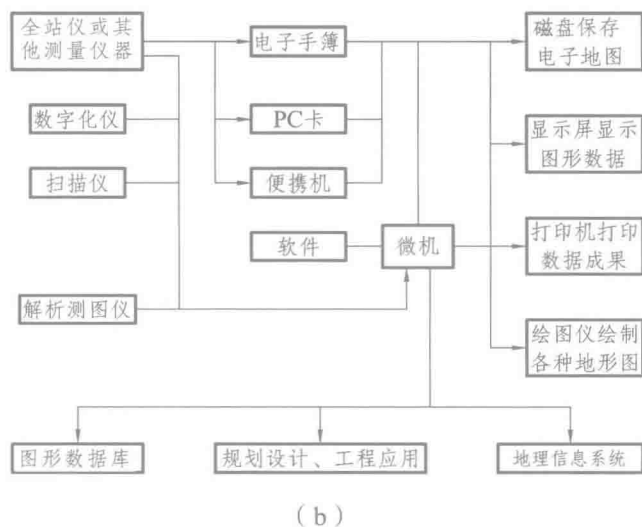
图 1-4 数字化测图系统硬件配置与连接方式
