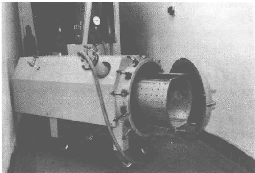
上海市档案局馆研制的真空充氮杀虫容器
