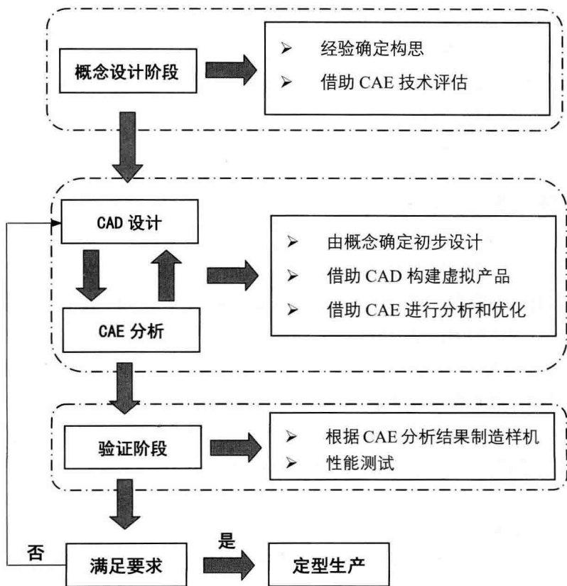
图 1.1.2 现代的产品设计流程图
