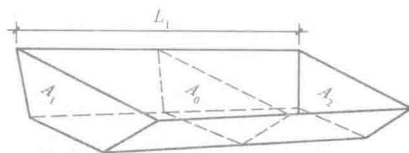
图 1-3 基槽土方量计算
