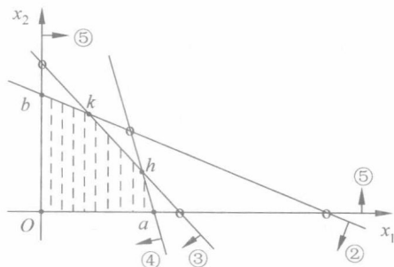
图 1-1 数学模型的可行解域
