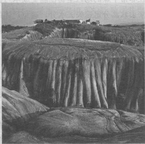
流动的岩层
