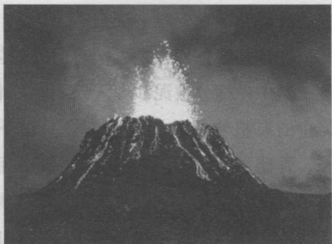
火山爆发
