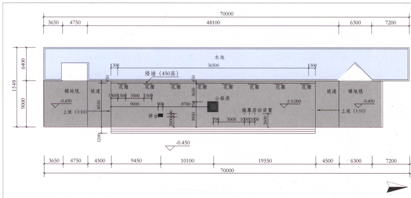
第二稿方案平面图
