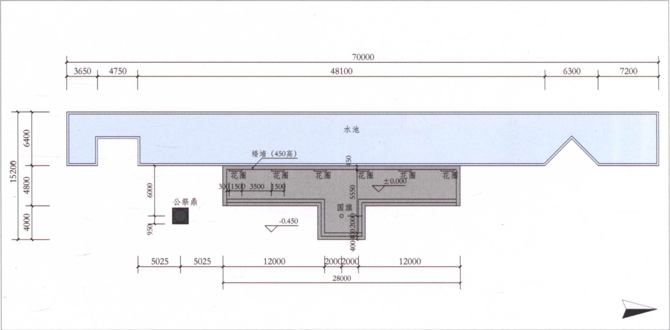
第一稿方案平面图
