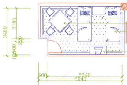
按摩包房平面布置图
