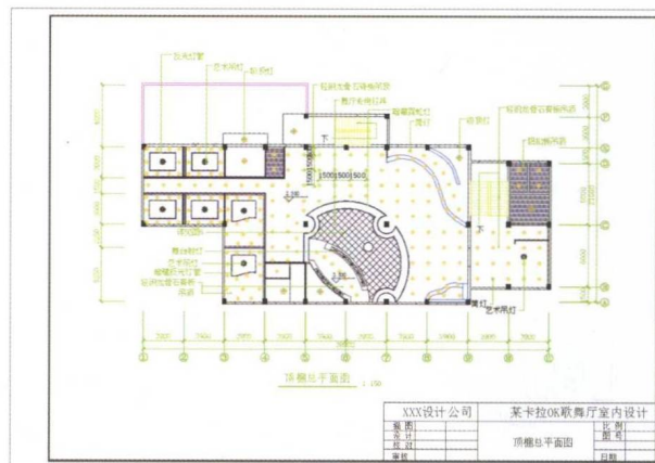
4.2.2 歌舞厅室内顶棚图绘制
