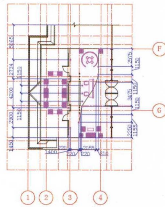
室内
