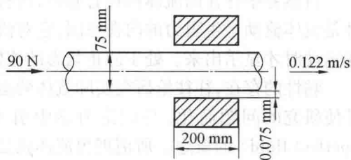
图1.2 轴与轴套
