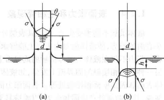
图 1.3 毛细管现象
