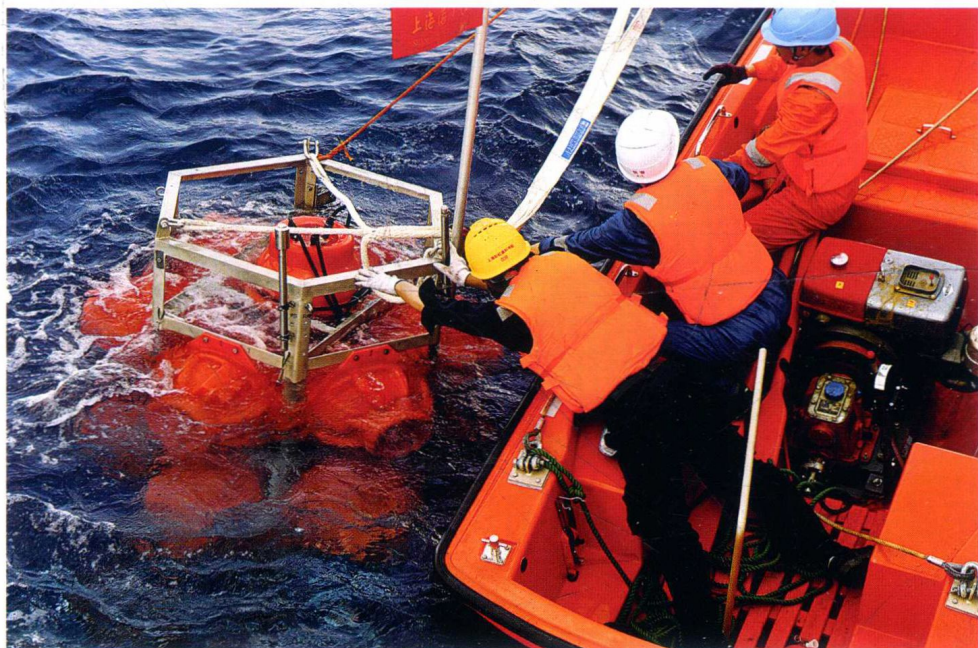
2016年7月18日,“张謇”号专用科考母船上的操作人员乘坐小艇回收着陆器。浩瀚美丽的南海,连日来风平浪静。自从7月17日抵达这片深蓝色目标海域,“张謇”号上的科考队员们就夜以继日,连续开展各项深海设备测试和科学考察,其中包括布放“彩虹鱼”万米级着陆器。
