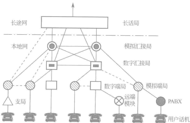
图 1-6 两级网的网络结构
