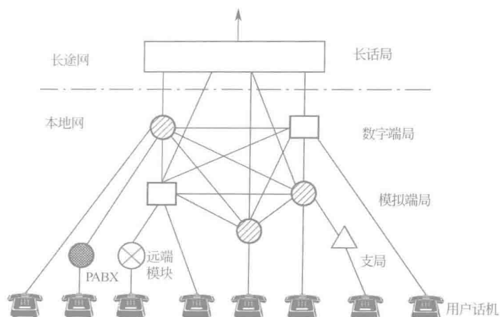
图 1-7 网型网结构
