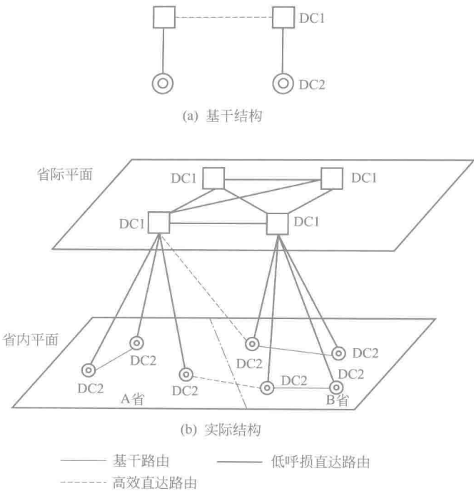
图 1-5 我国长途网的两级网络结构
