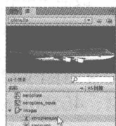
图 10-2-2 导入到库
