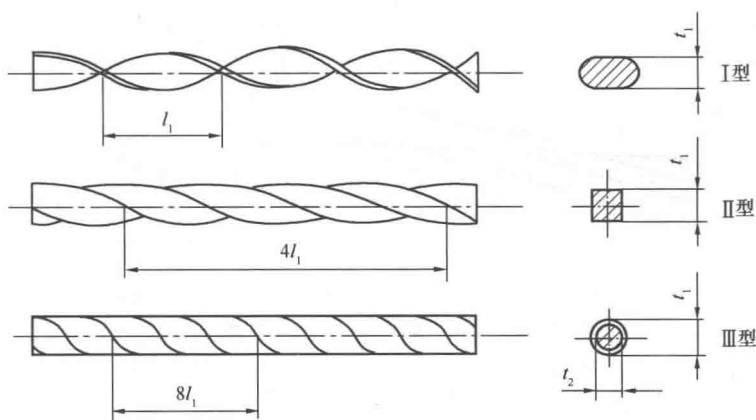
图 1-3 冷轧扭钢筋形状及截面控制尺寸
