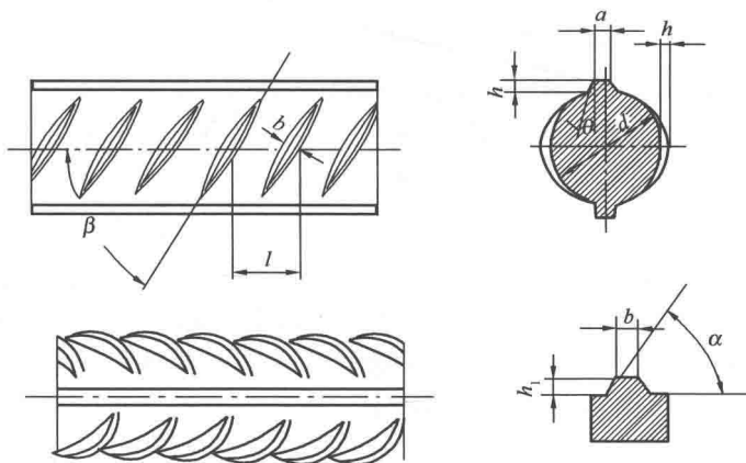
图 1-1 月牙肋钢筋表面及截面形状
