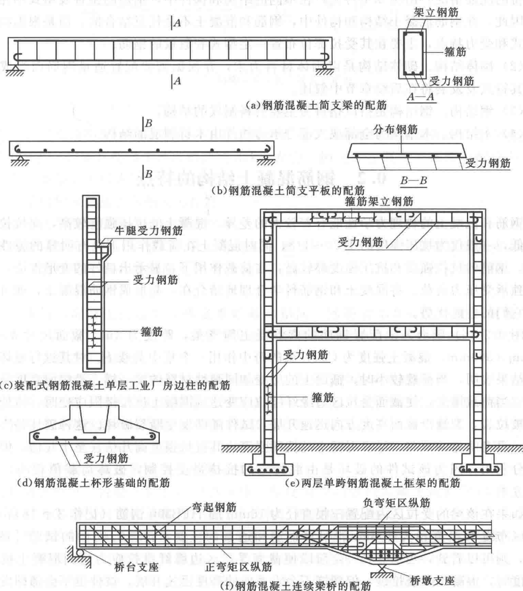
图 0.1 常见钢筋混凝土结构和构件配筋实例
