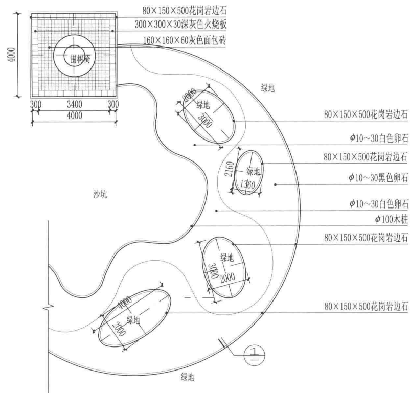
卵石路面平面图
