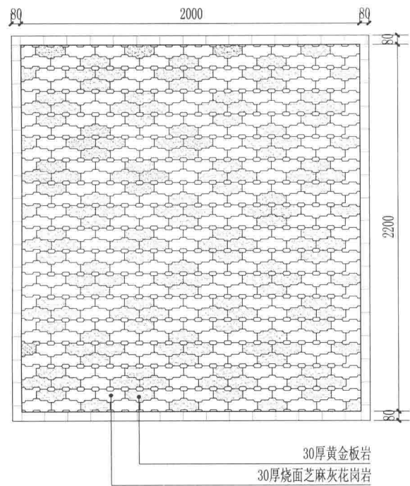
花街铺装样式 (1)
