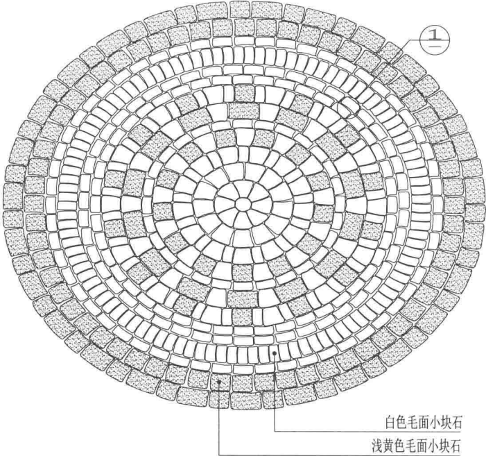
花街路面平面图
