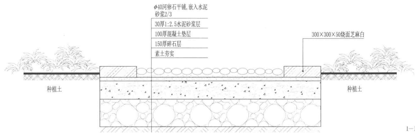
1-1剖面图
