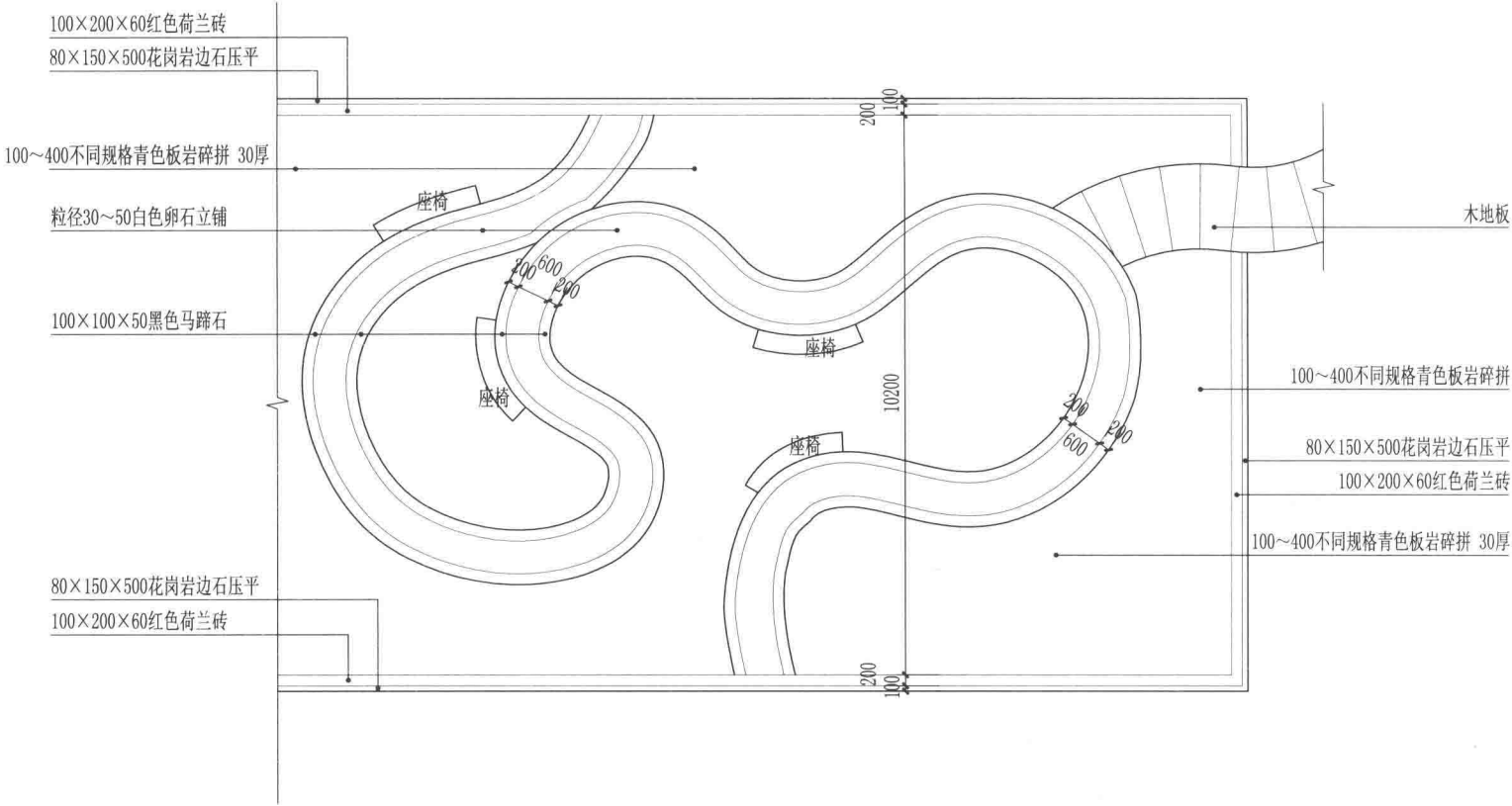
卵石路面平面图
