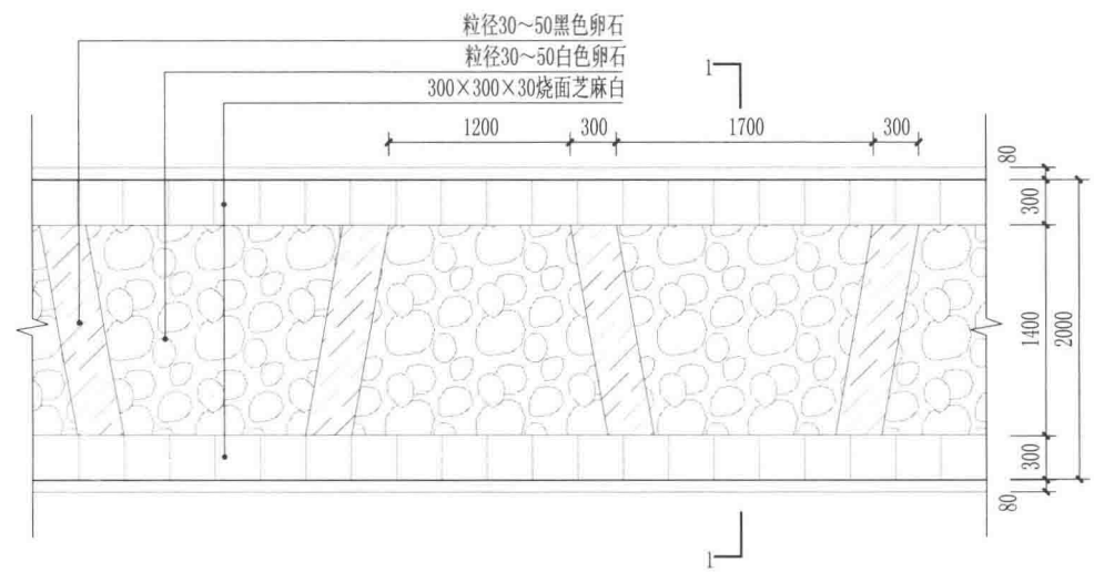
卵石路面平面图
