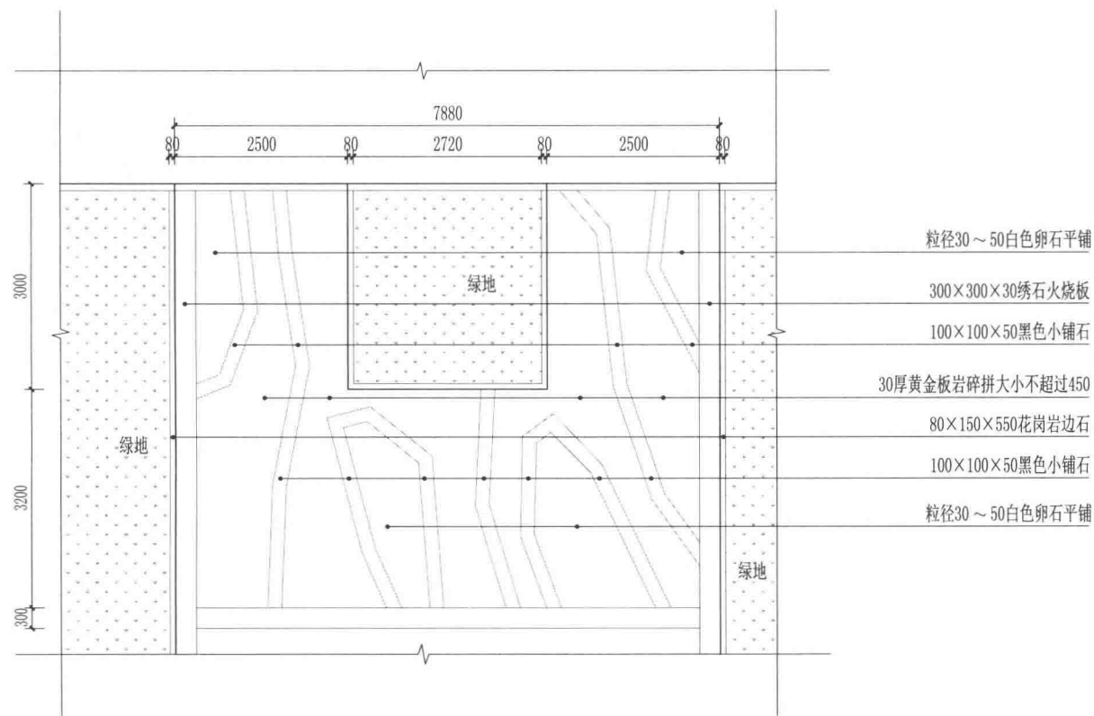
卵石路面平面图
