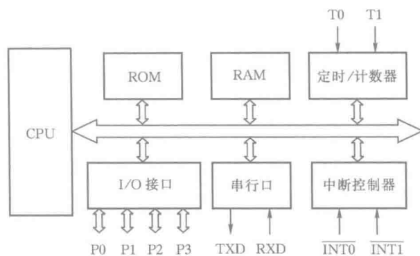
图 2.1 MCS-51 系列单片机的内部结构
