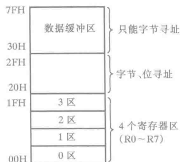
图 2.3 内部 RAM 结构
