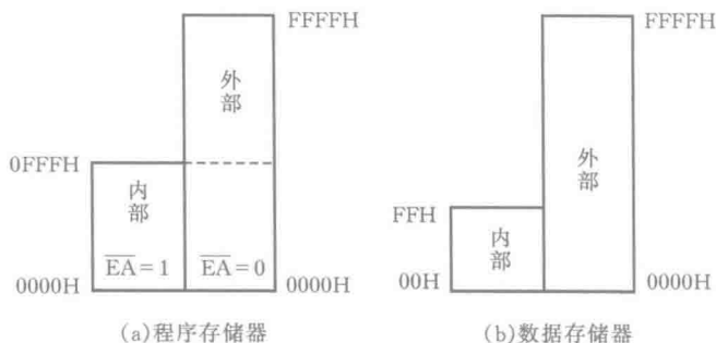
图 2.2 MCS-51 存储器空间
