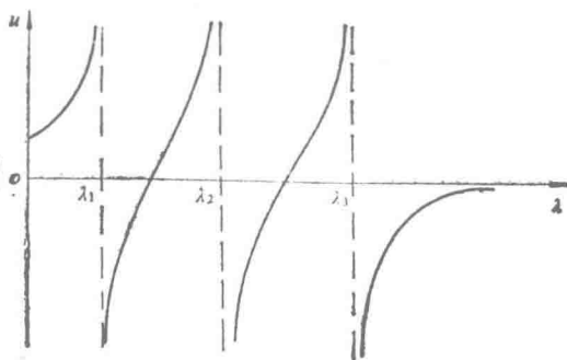
(a) 无刚体自由度, 无纯静态自由度
