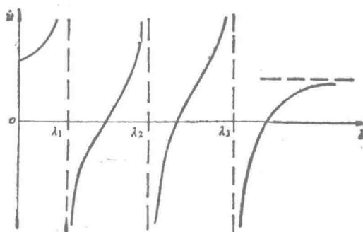
(c) 无刚体自由度, 有纯静态自由度
