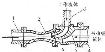
图 1-11 喷射泵
