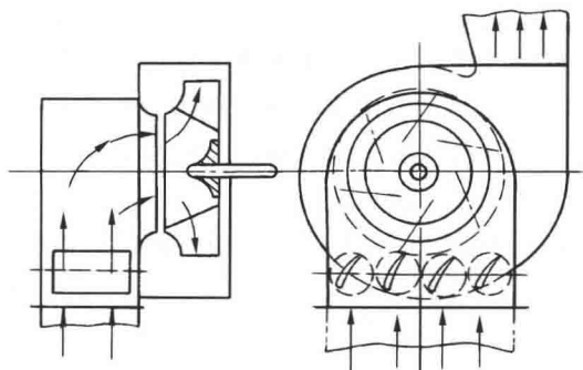
图1-3 离心风机
