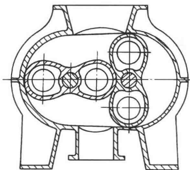
图 1-8 罗茨鼓风机
