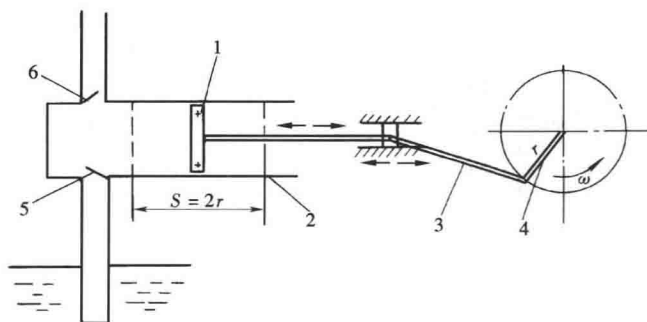
图 1-6 活塞泵
