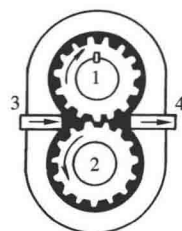
图 1-7 齿轮泵
