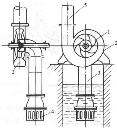
图 2-2 离心式水泵
