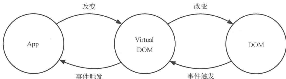
图 1-2 React DOM 更新
