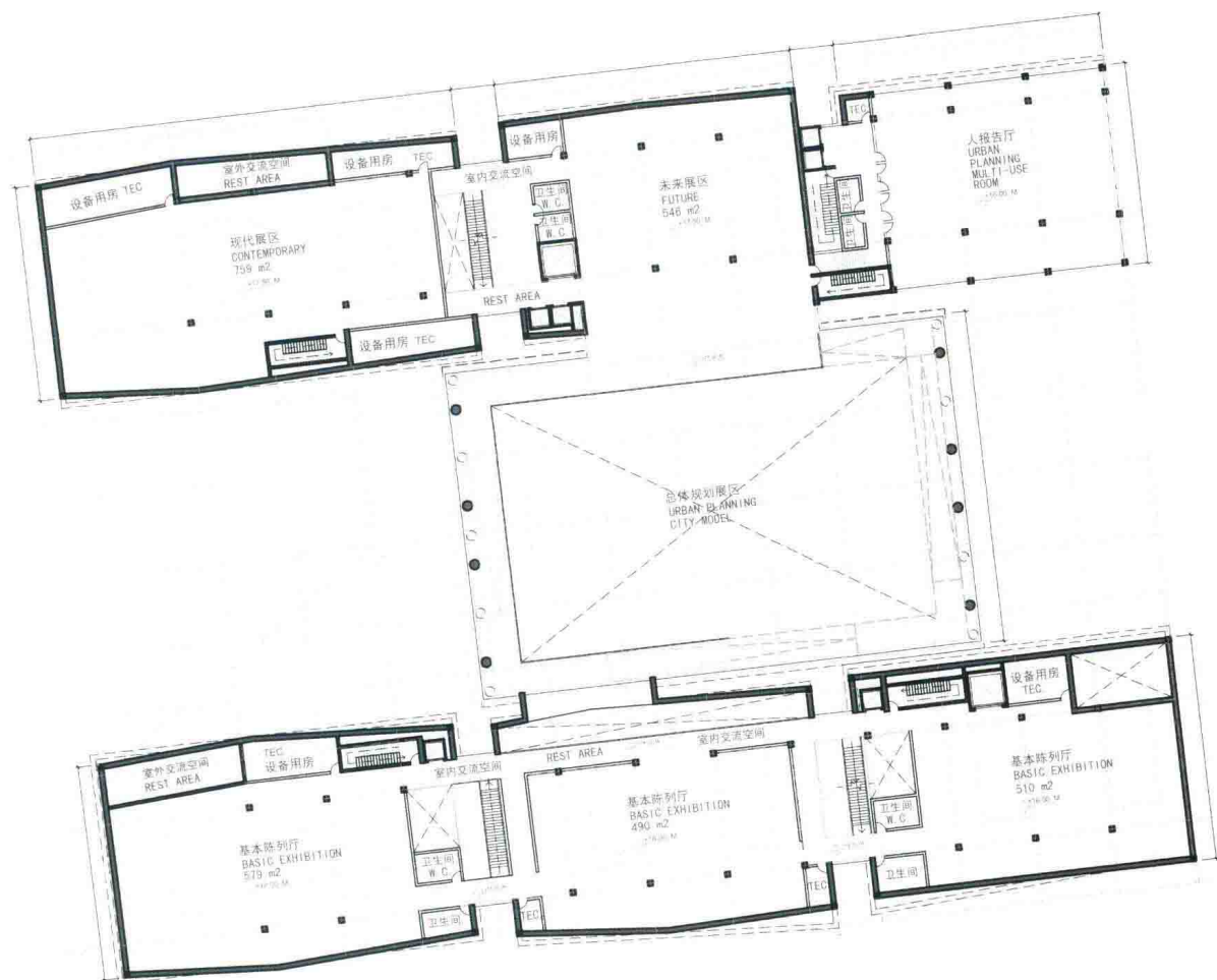
四层平面图
