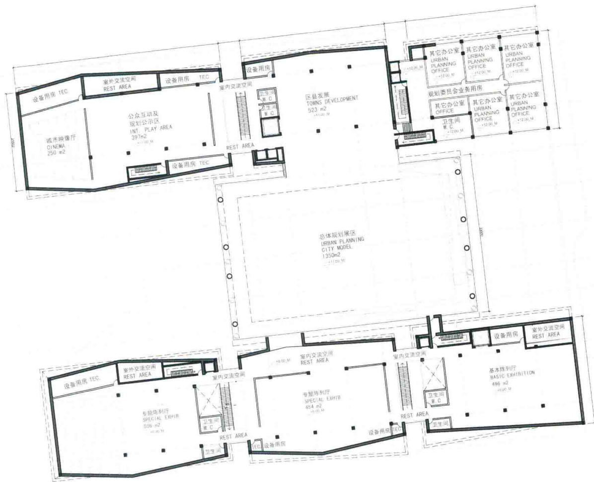
三层平面图
