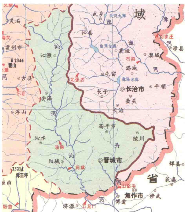
图1. 沁河流域山西区域水系示意图
