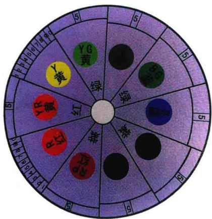
彩图 13 10 色色相环
