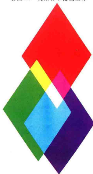
彩图 20 色彩的加光三原色
