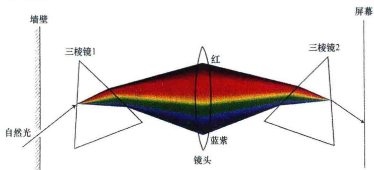
彩图1 可见光波示意图
