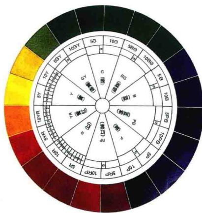
彩图 14 12 色色相环
