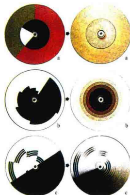
彩图 22 色彩的旋转混合
