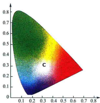
彩图 19 CIE、XYZ 系色度坐标
