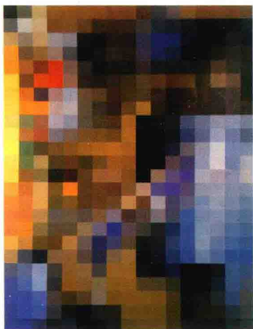
彩图 23 色彩的空间混合图形
