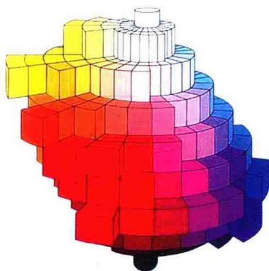
彩图 17 孟塞尔色相树
