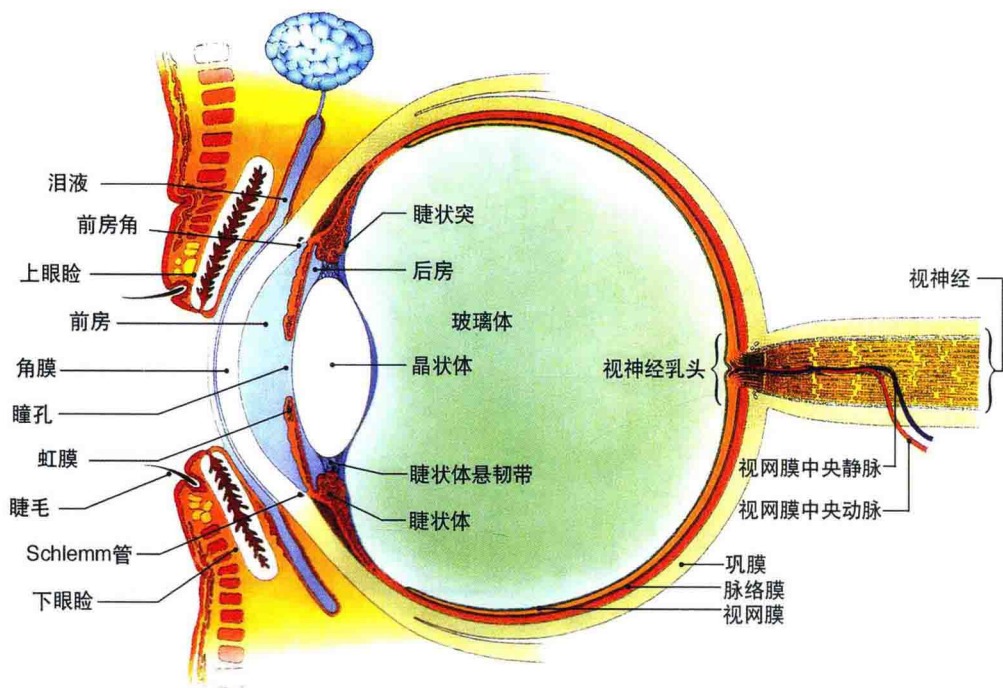
彩图 7 眼睛构造示意图
