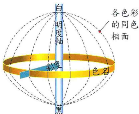
彩图 9 色立体原理构造图
