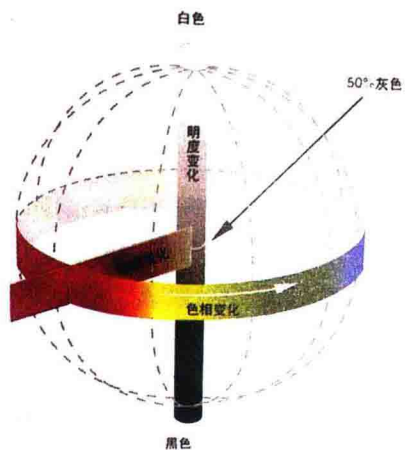
彩图 16 色立体模型示意图
