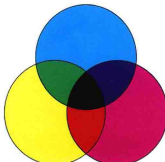
彩图6 色彩三原色
