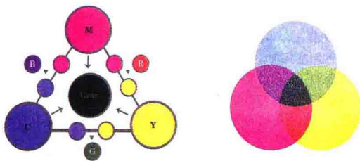
彩图 21 颜料三原色减法混合
