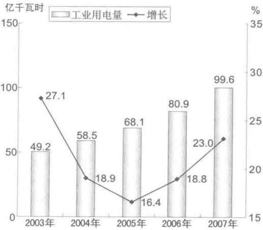
图9 2003—2007年工业用电量及其增长速度
