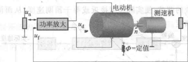
图 1-11 闭环控制的调速系统
