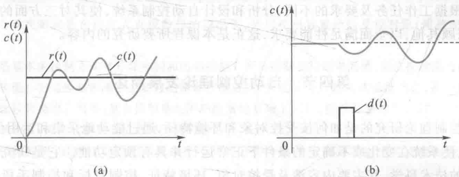
图 1-14 不稳定恒值系统的动态过程
