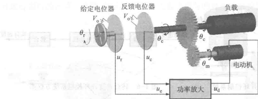
图 1-9 位置随动系统
