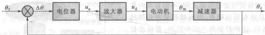
图 1-10 位置随动系统方框图
