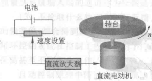
图 1-5 转台速度开环控制系统
