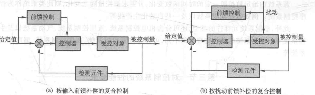
图 1-12 复合控制方式
