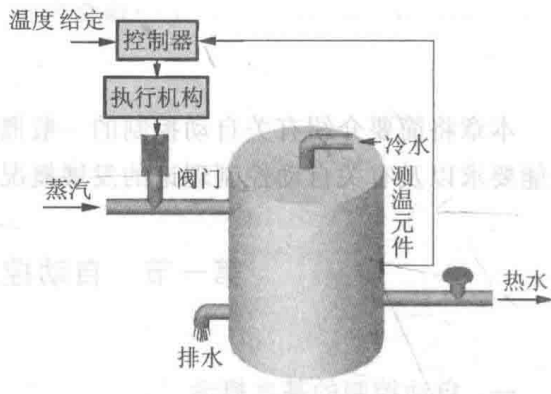
图 1-3 水温自动控制系统
