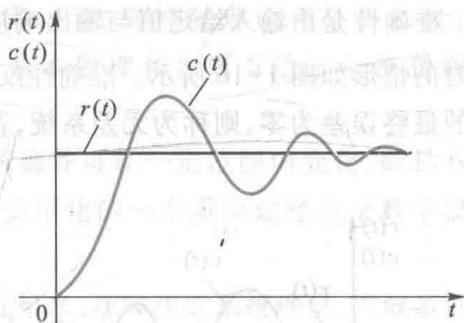
图 1-13 稳定恒值系统的动态过程
