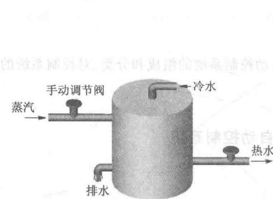
图 1-2 水温人工控制系统
