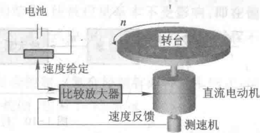
图 1-7 转台速度闭环控制系统
