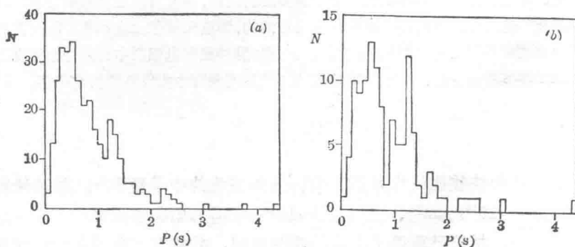
图1. 射电脉冲星的周期分布的直方图。
