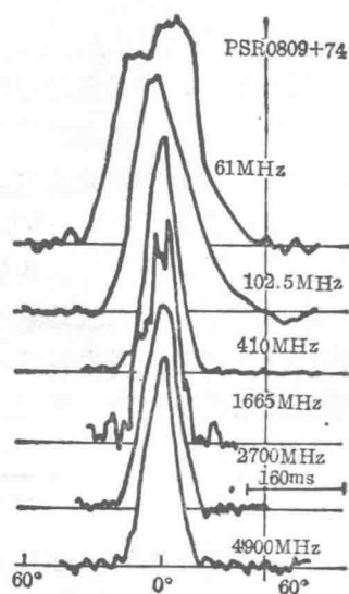
图4. PSR 0809+74的积分脉冲轮廓随观测频率的变化 [27] 。
