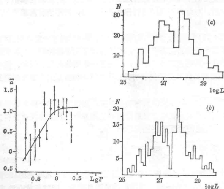
图2. 平均谱指数 \bar{\alpha} (在102—408MHz)对脉冲星周期的依赖关系 [15] 。
