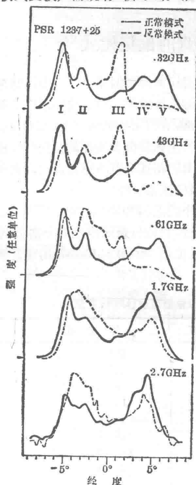
图 7. PSR 1237+25 在不同频率下的脉冲轮廓。正常模式是 1 000 次脉冲的平均,而反常模式是 100 次的平均 [29] 。
