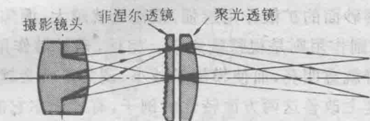
图 2 菲涅尔透镜和聚光透镜
