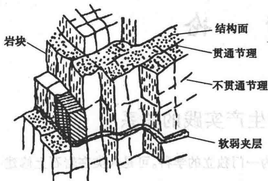
图 1.1 岩体结构示意图
