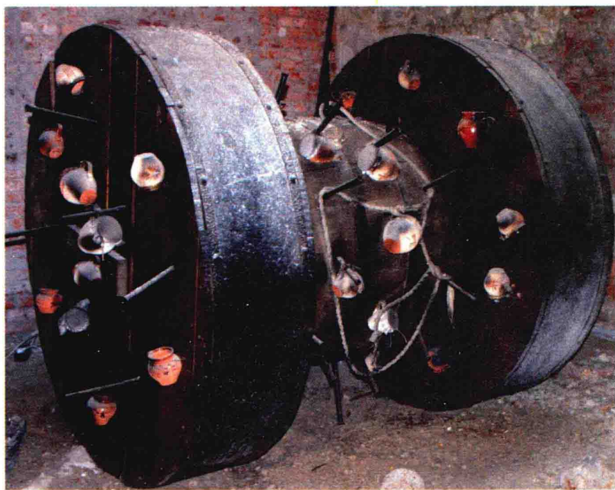
盖尔盖义发明制造的射击火轮
