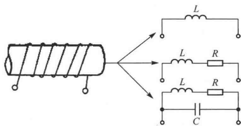
图 1.3 实际电感的不同模型
