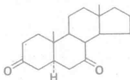
5 \alpha -Androstane-3, 7-dione
